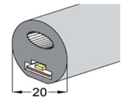
MOD. R023 D20 mm PCB 10 mm
