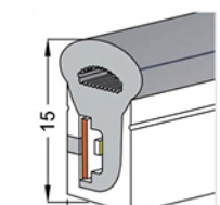
MOD. V016 8x15 mm PCB 5 mm
