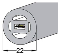
MOD. R037 D22 mm PCB 5 mm
