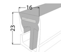
MOD. V055 16x24 mm PCB 10 mm
