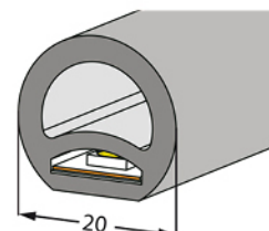
MOD. R000 D20 mm PCB 10 mm
